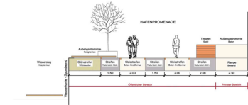
Systemschnitt Hafenpromenade M 1:100
