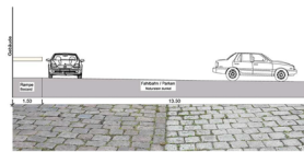
Regelquerschnitt Bestand M 1:100
